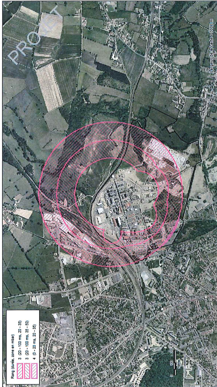
PPRT de Commentry (ADISSEO) Phénomènes dangereux de référence dans la zone 20 - 50 mbar
