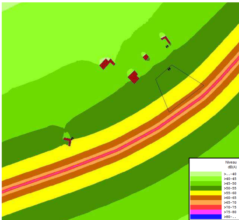
Figure 4 : Cartographie sonore hauteur = 2 m – Bruit Résiduel – Nuit
