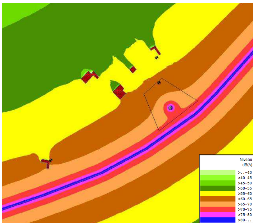
Figure 5 : Cartographie sonore hauteur = 2 m – Bruit Ambiant – Période Jour
