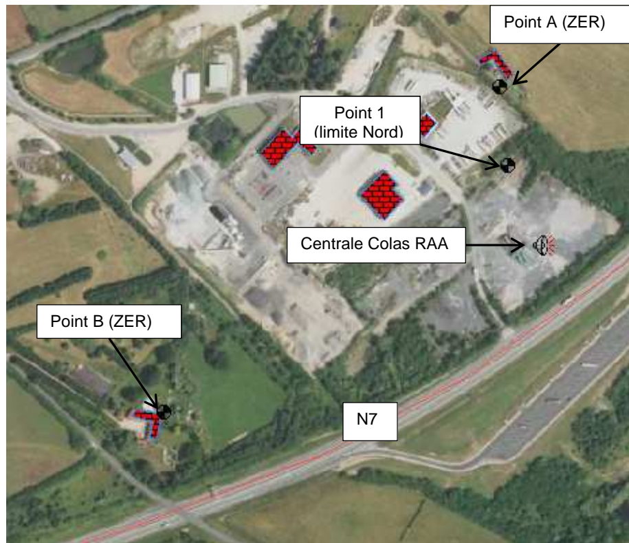
Figure 2 : Vue en plan du modèle informatique de prévision IMMI
