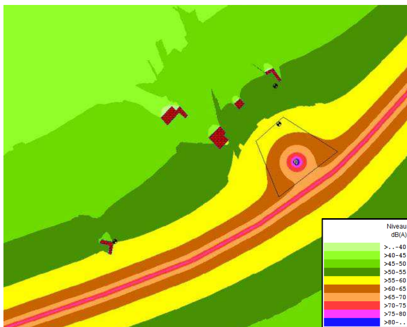
Figure 6 : Cartographie sonore hauteur = 2 m – Bruit Ambiant – Période Nuit
