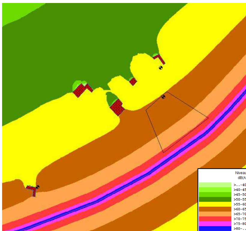
Figure 3 : Cartographie sonore hauteur = 2 m – Bruit Résiduel – Jour
